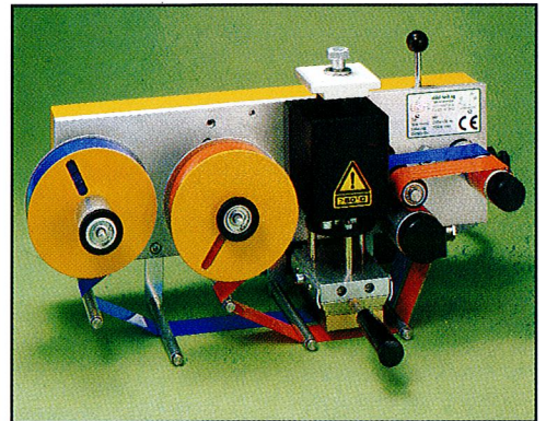
dübi-tech Printer für zwei separate Prägefolien
