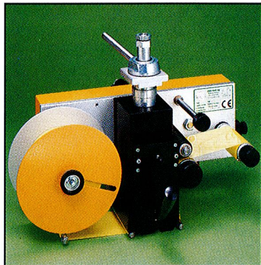
dübi-tech Printer mit 1000 m Folienrolle und Hubfeineinstellung
