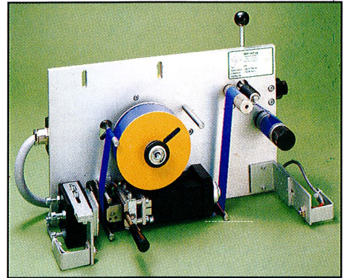
Laschencodiergerät für aufgerichtete Schachtelzuschnitte, Siegel- und Falzverschlüsse
