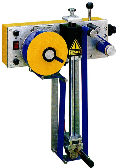
dübi-tech Printer mit verlängerter Kolbenstange für schlecht zugängliche Druckpositionen.
